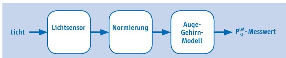
Bild 2: Blockschaltbild P_{st}^{LM} -Messverfahren
